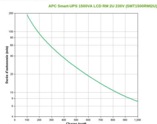
Diagramme d'autonomie
