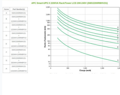
Diagramme d'autonomie
