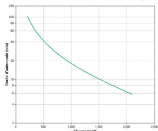
Diagramme d'autonomie
