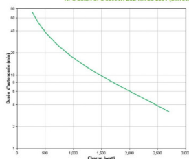
Diagramme d'autonomie
