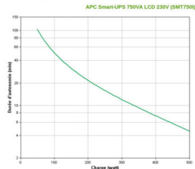
Diagramme d'autonomie
