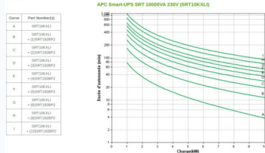
Diagramme d'autonomie
